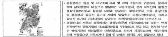
라. 지체구조
